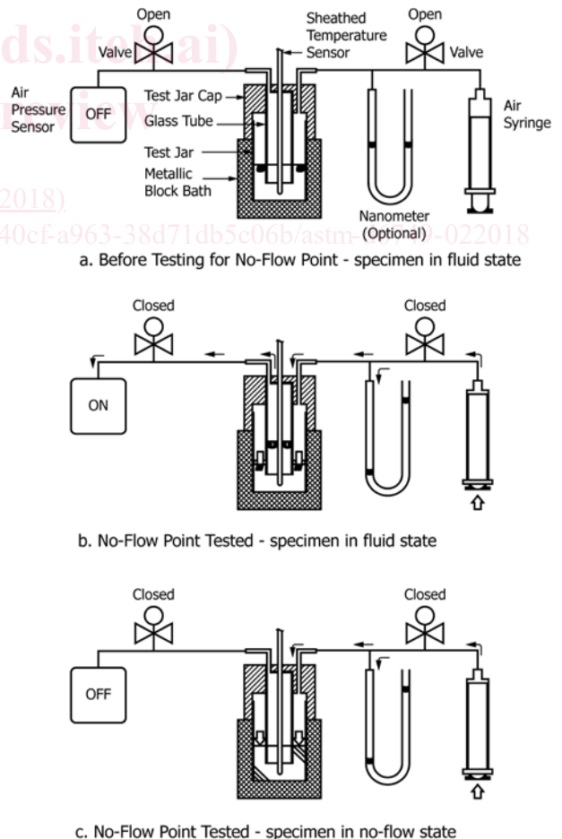
FIG. 1 Automatic Apparatus
