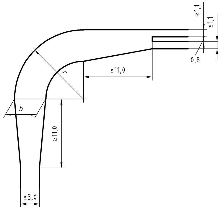
Bild 3 — Nicht geradlinig geführte Zufahrt
