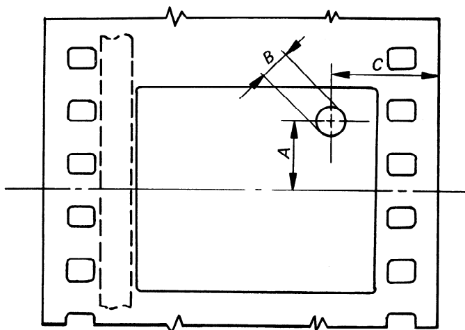
Figure 2 — Emplacement des marques « moteurs » et des marques de « passage »
