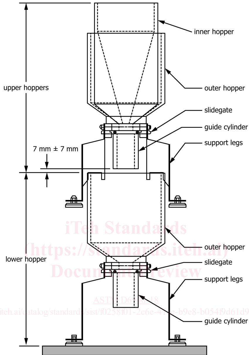
FIG. 1 Apparatus
