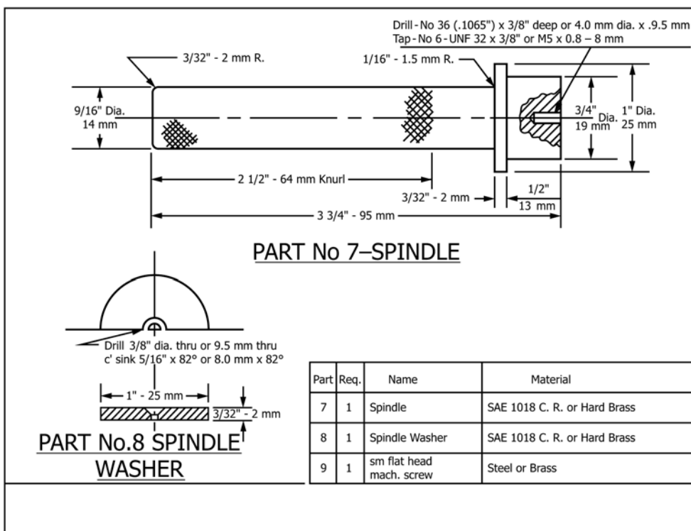
FIG. 4 Spindle
