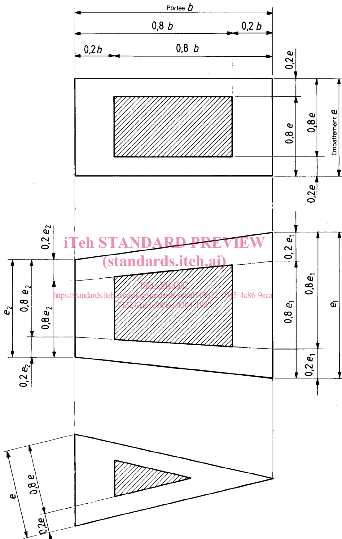
Figure — Configurations de la base des appareils de levage
