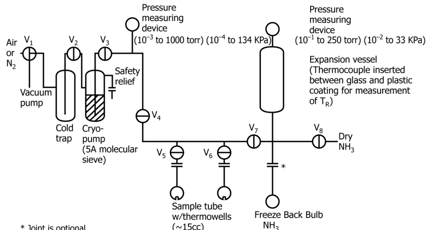
FIG. 1 Apparatus
