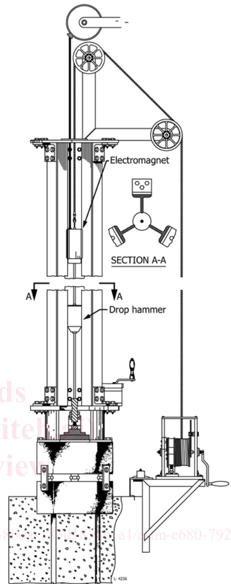
FIG. 3 U.S. Bureau of Mines Impact Apparatus
