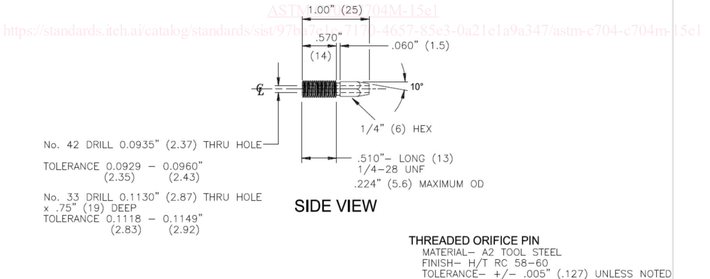
FIG. 4 Venturi Nozzle
