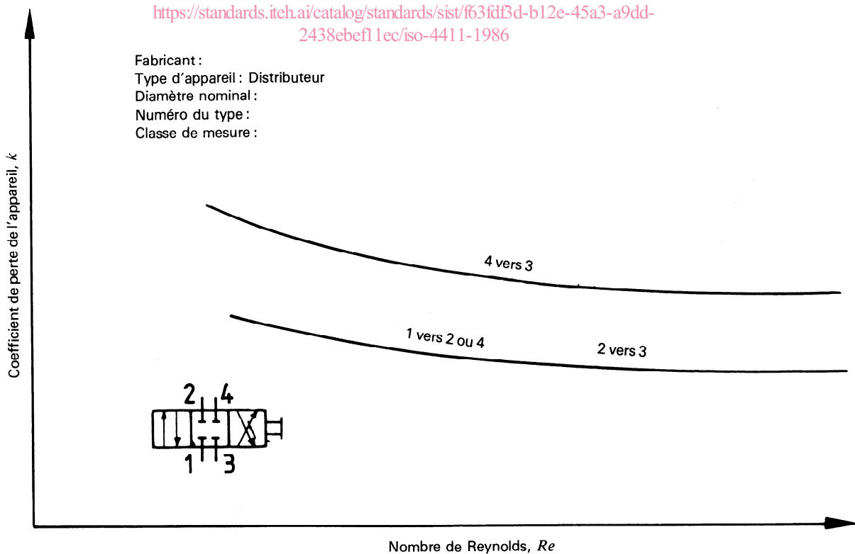
Figure 2 — Présentation sans dimensions d'un distributeur
