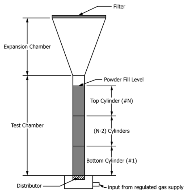
FIG. 1 Apparatus
