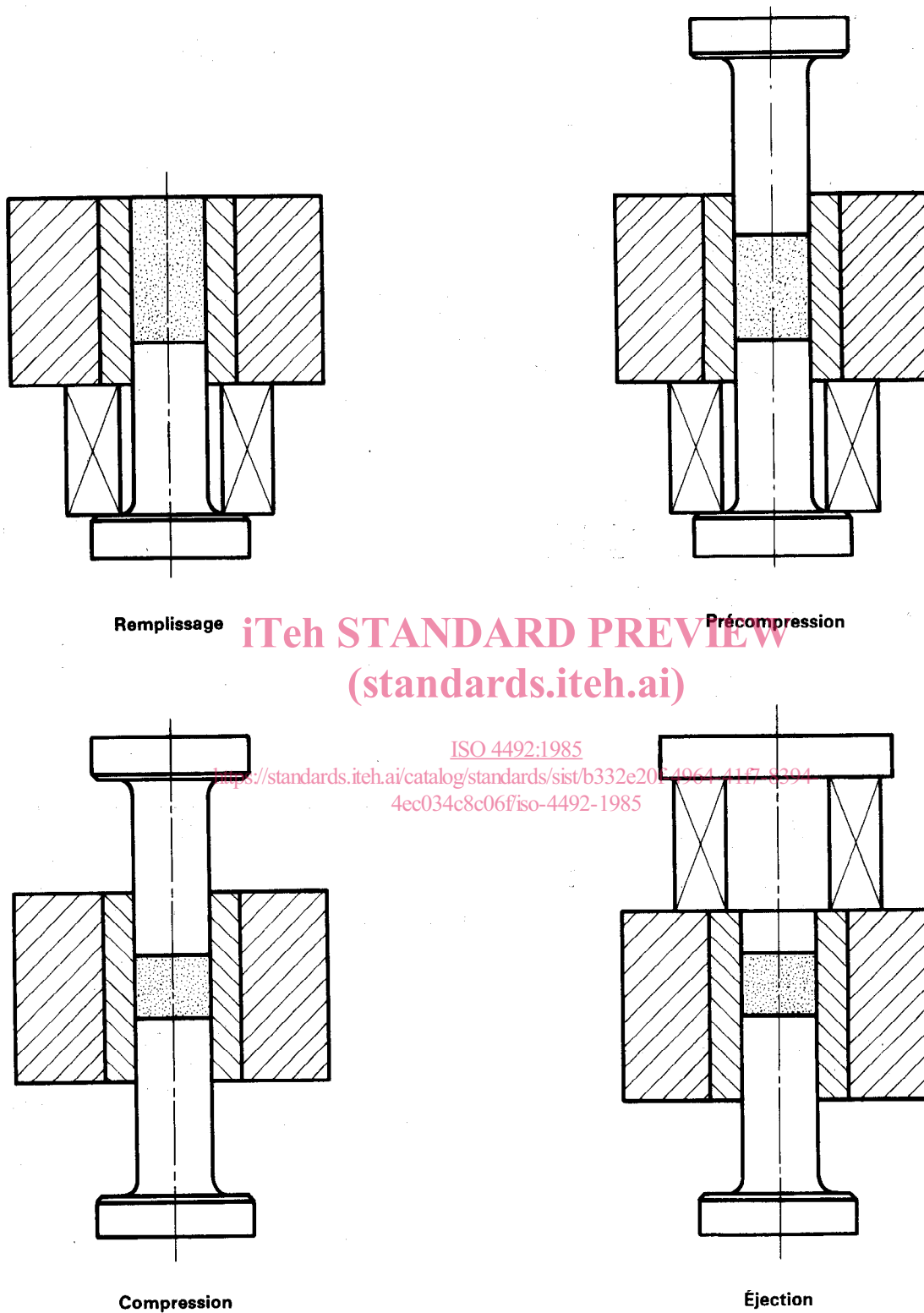
Figure 3 – Schéma de production d'un comprimé
