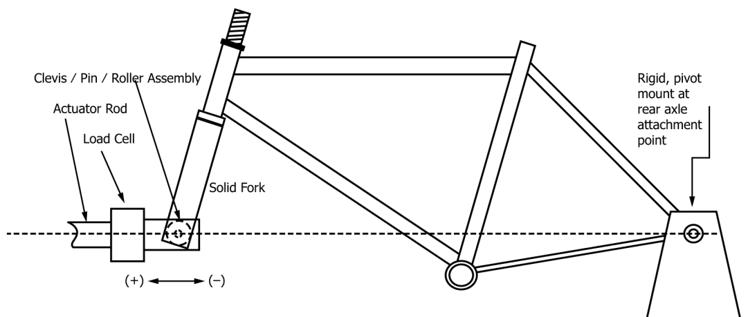
FIG. 1 Horizontal Fatigue Test
