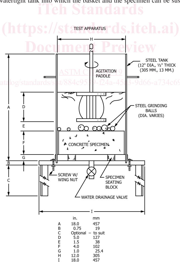
FIG. 1 Test Apparatus
