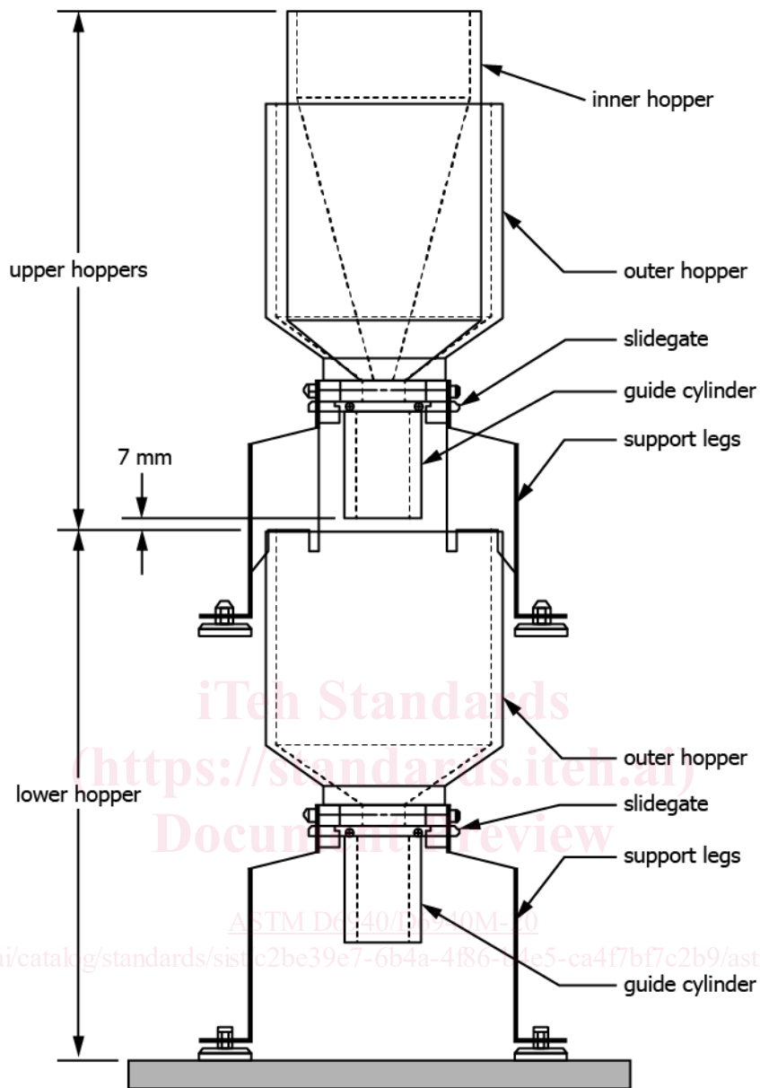
FIG. 1 Apparatus
