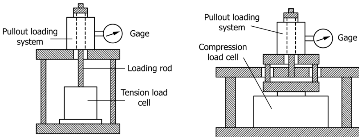
(c) Calibration using tension load cell (d) Calibration using compression load cell
