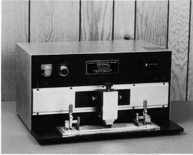
FIG. 1 Granule Adhesion Test Apparatus
