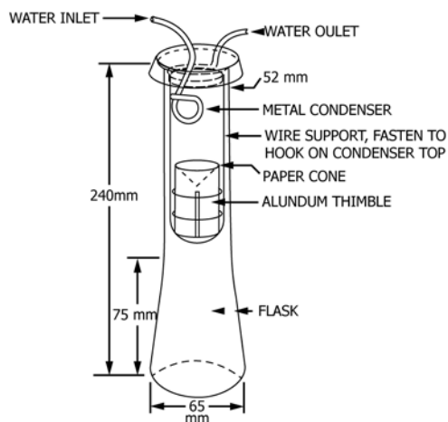
FIG. 1 Extraction Apparatus
