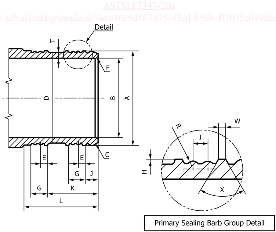
FIG. 1 Metal Insert Dimensions
