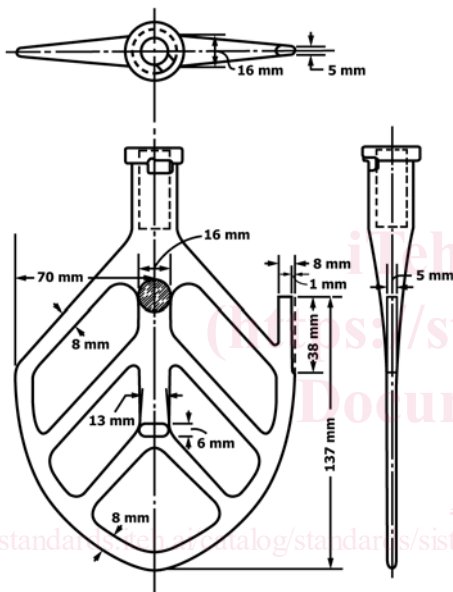
FIG. 2 Paddle
