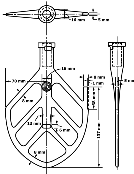
FIG. 2 Paddle
