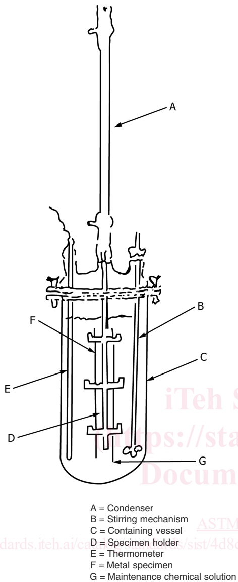
FIG. 1 Test Apparatus
