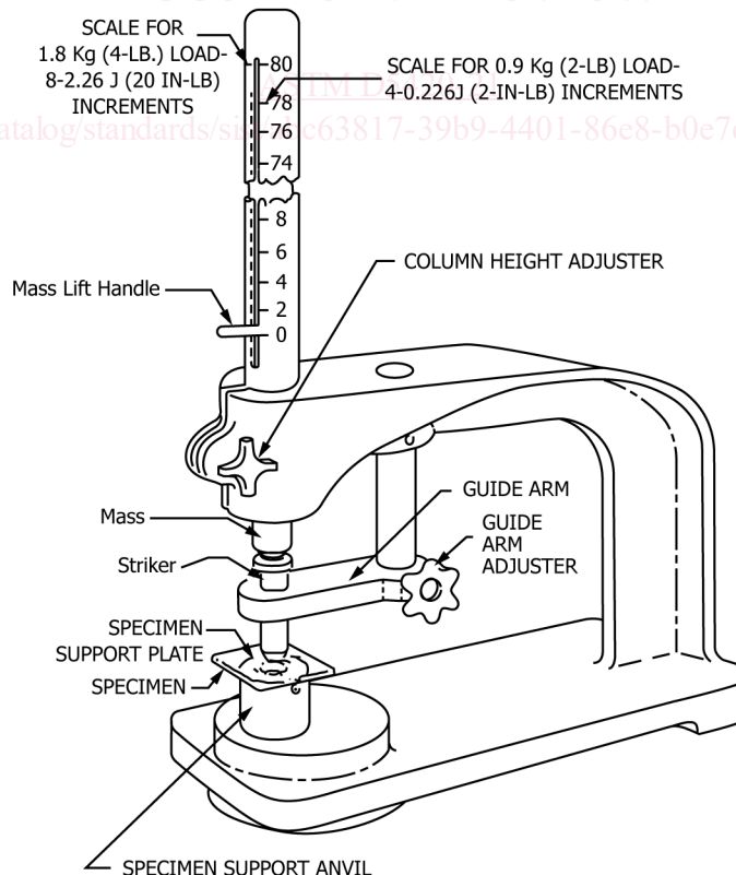
FIG. 1 Impact Tester
