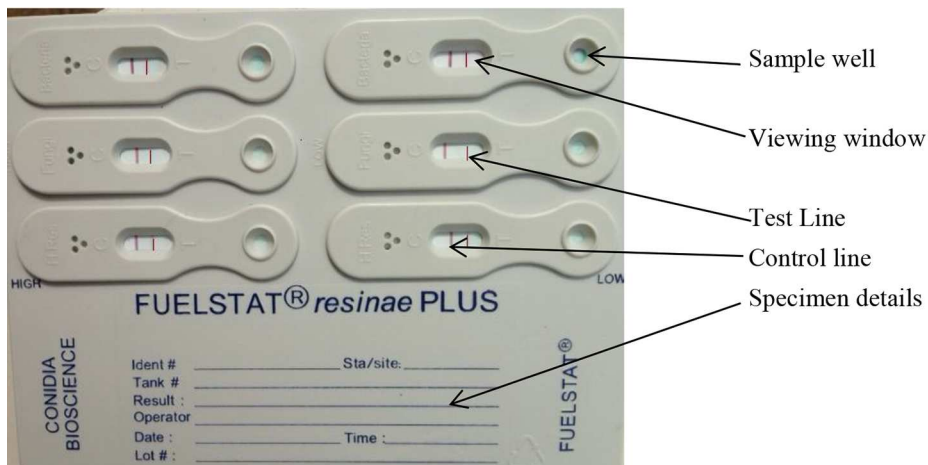
FIG. 2 LFD Tray
