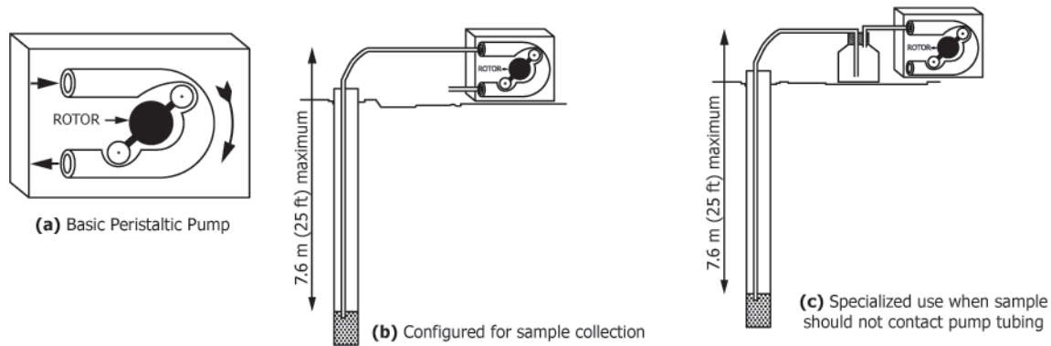
Peristaltic Pump FIG. 1 Peristaltic Pump
