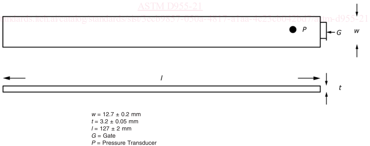
FIG. 3 Bar Specimen
