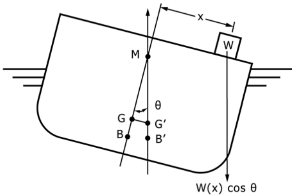
FIG. 2 Metacentric Height
