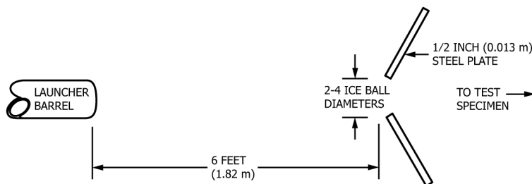
FIG. 4 Sabot Trap
