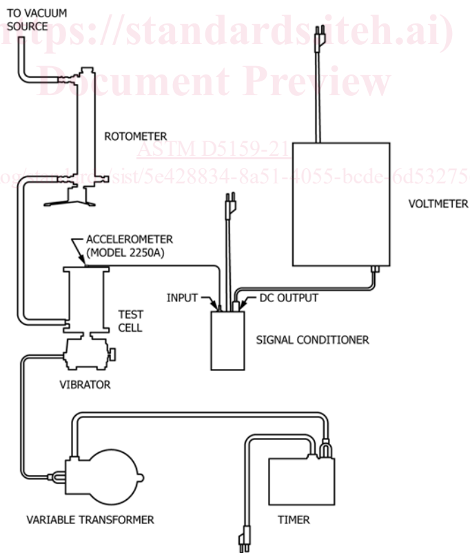
FIG. 2 Apparatus Assembly
