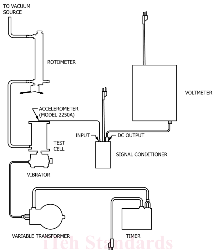
FIG. 2 Apparatus Assembly
