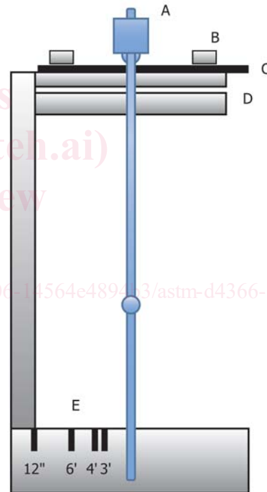
FIG. 2 Apparatus Manual Type
