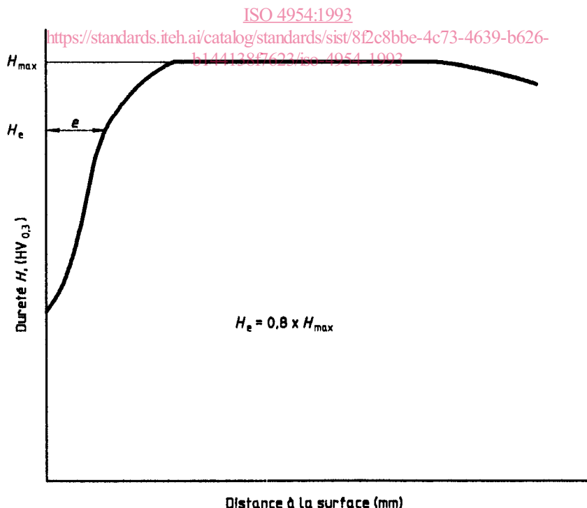
Figure 1 — Détermination de la profondeur de la zone décarburee
