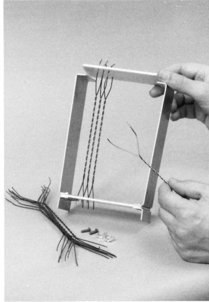
FIG. 4 A-Specimen Holder
