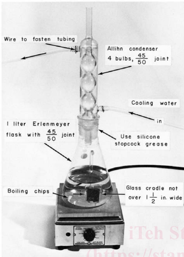
FIG. 1 Test Apparatus
