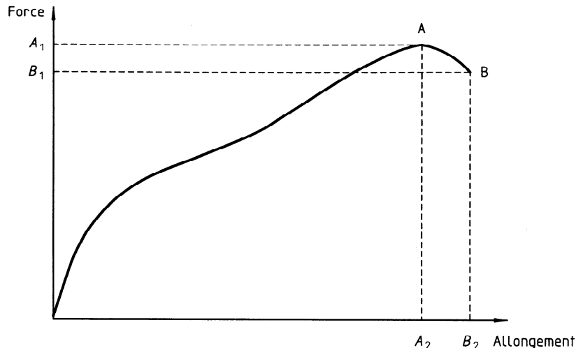
Figure 1 — Courbe type force/allongement
