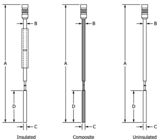
FIG. 1 D2983 Spindles
