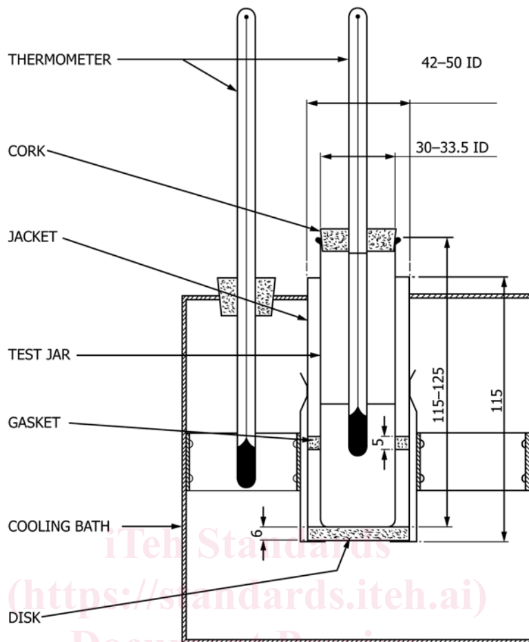
FIG. 1 Apparatus for Pour Point Test
