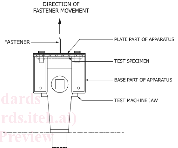
FIG. 2 Apparatus
