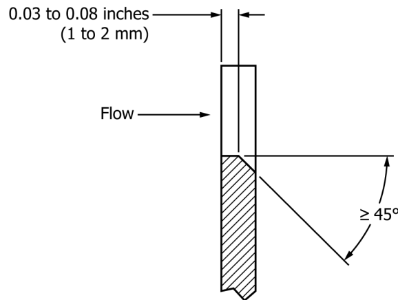
Notch edge section (A-A).
