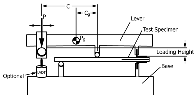
FIG. 1 MMB Apparatus
