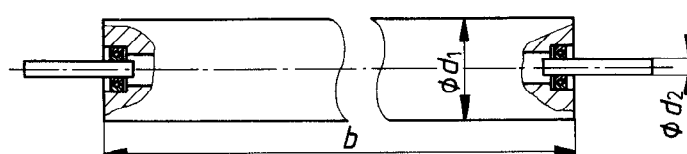
Figure 2 — Type B: Rouleau à axes fixes
