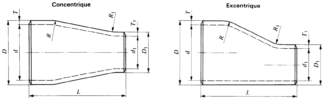
Figure 4 – Réductions concentriques et excentriques (standards.iteh.ai)
