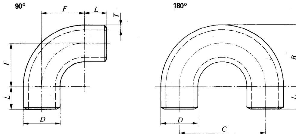
Figure 2 – Courbes 3D (avec parties droites)
