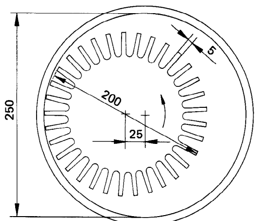
Figure — Éléments principaux du moulin PFI
