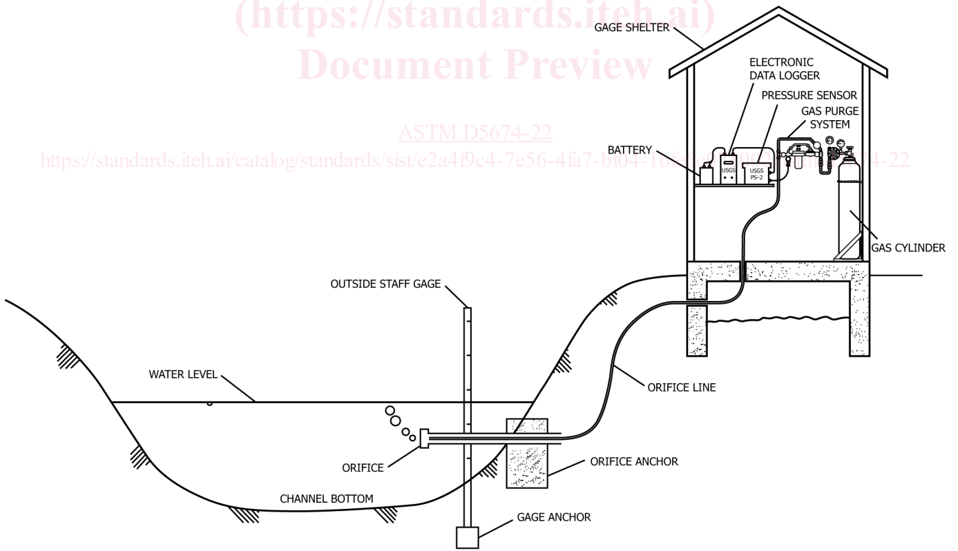
FIG. 2 Bubble Gage
