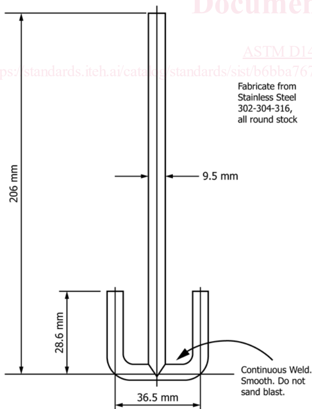
FIG. 2 Stirrer
