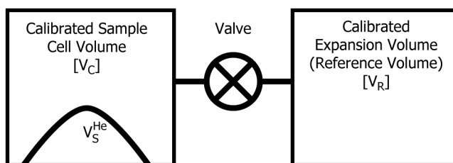
FIG. 2 Pycnometer Apparatus
