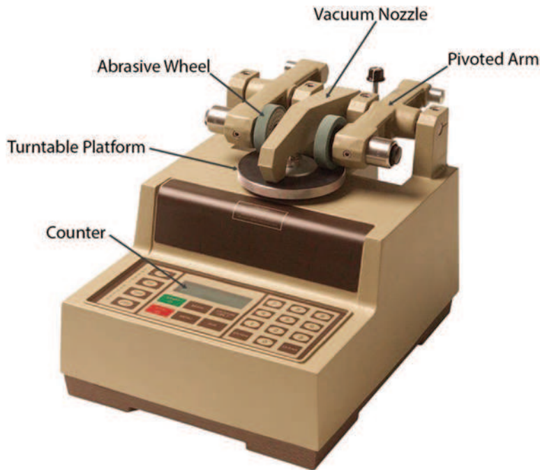
FIG. 1 Taber Abraser
