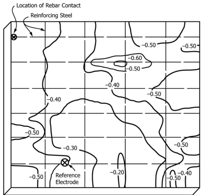
FIG. 3 Equipotential Contour Map
