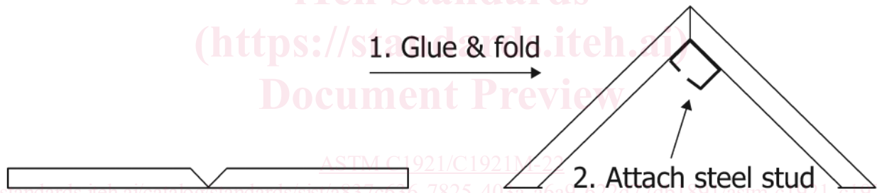
FIG. 4 Mitred Corner
