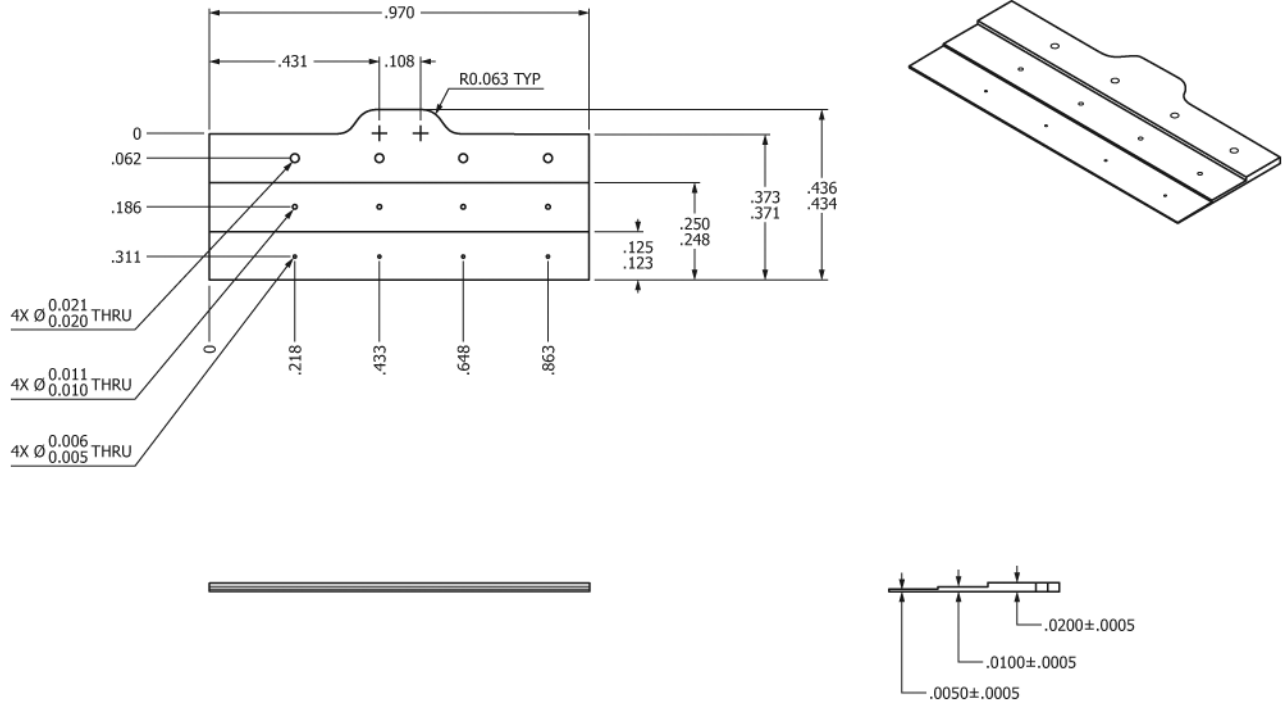
FIG. 4 Shim
